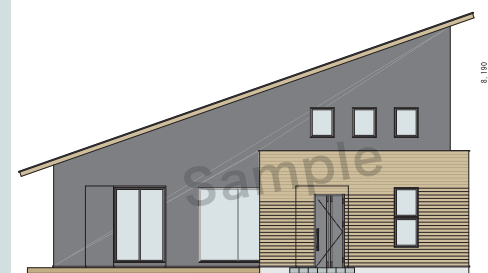
立面
