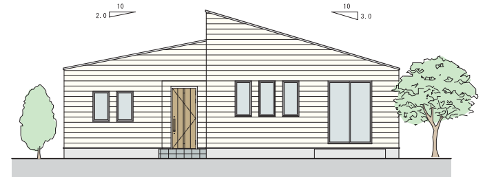
南側立面図 S=1:100
